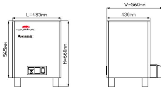
OCS-90B
